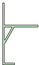
Art.2310 Sostegno a parete Wall bracket
