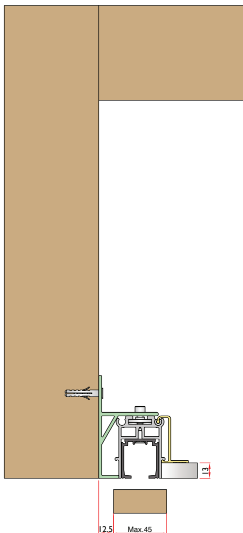
Sistema per fissaggio a parete Wall-mounting system
