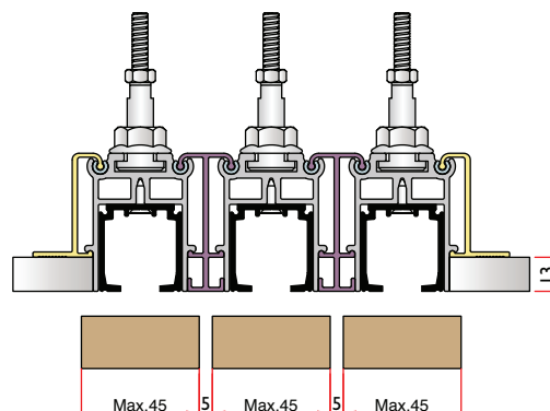
Regolazione superiore Top adjustment
