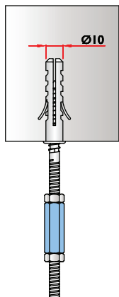
Sistema per fissaggio soffitto vuoto Empty ceiling fixture system
