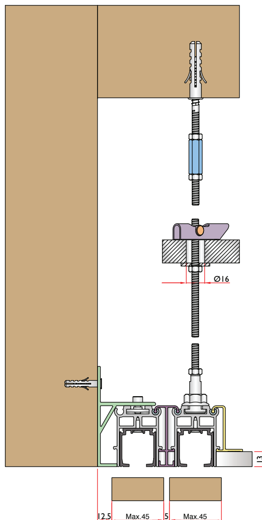
Sistema per fissaggio a parete e soffitto Wall and ceiling mounting system
