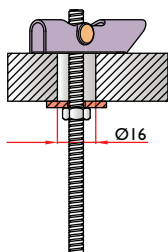
Sistema per fissaggio soffitto vuoto Empty ceiling fixture system
