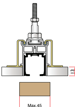
Regolazione sostegno inferiore Adjustment lower support
