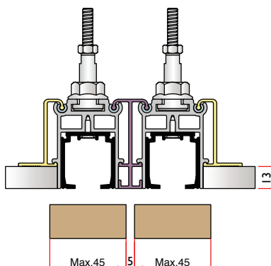
Bloccaggio dado Locking nut
