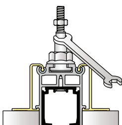
Regolazione sostegno inferiore Adjustment lower support
