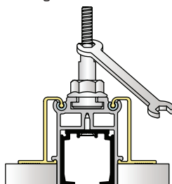
Bloccaggio dado Locking nut
